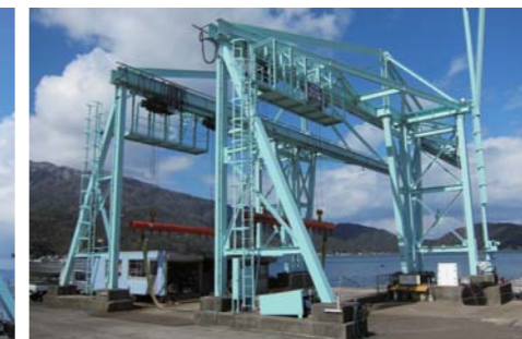
マリーナ内には大型の60フィートガントリークレーンが完備されており、小型艇~大型艇までオーナーの大切なボートを安心・安全に揚降してくれる。 取材協力:ファーストハーバーツルガ 福井県敦賀市名子37-19-1 TEL:0770-22-8777 URL:http://f-h-tsuruga.main.jp/
